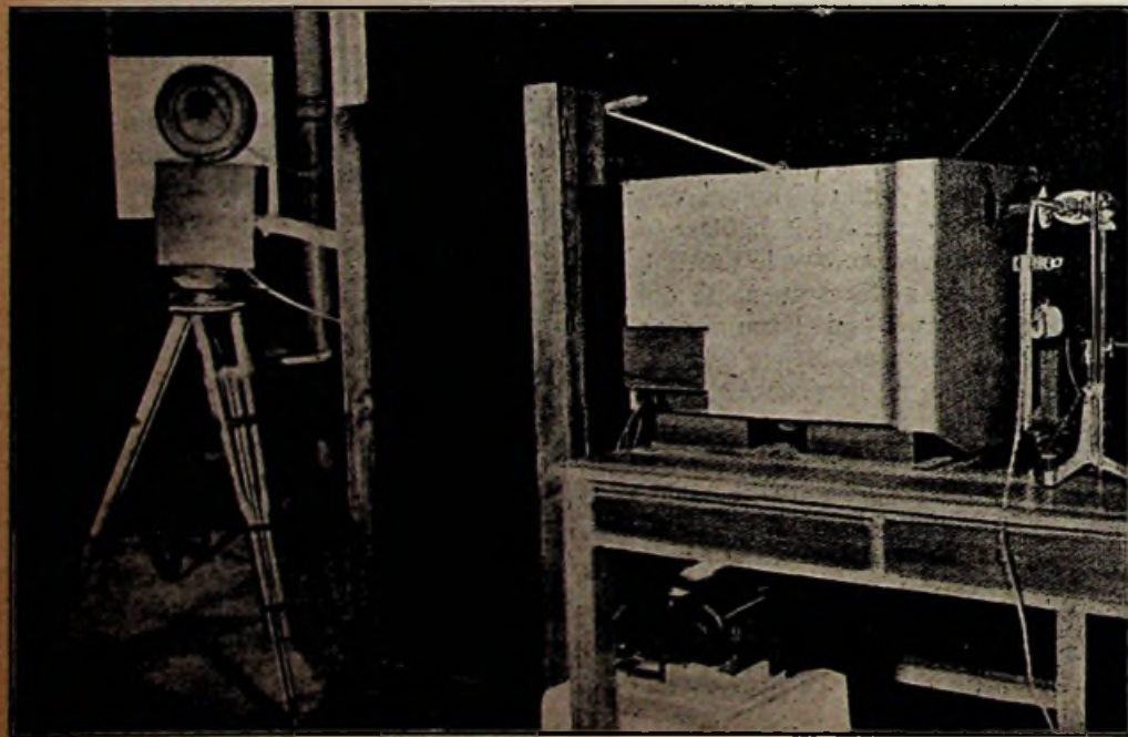
Fig. III. Laboratorium-uitvoering van den televisie-zender met filmfotografisch tussenprocedé.
